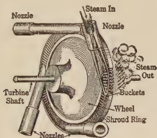
FIG. 177.—De Laval Nozzles, Blades and Disc.
